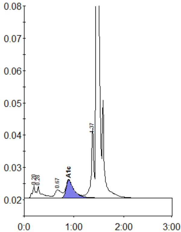
Peak table - ID: 10344453
